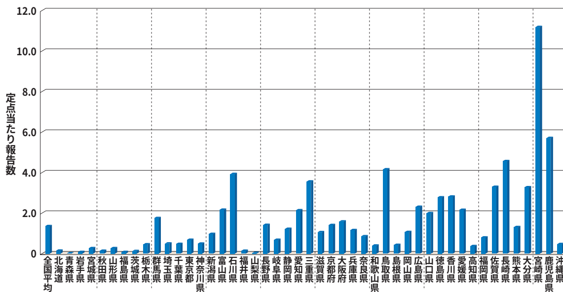
図2. 手足口病の都道府県別報告状況(2008年第24週)
